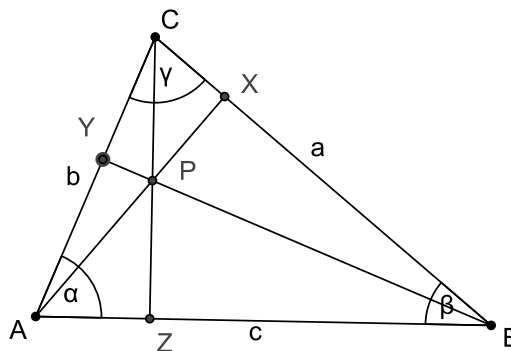
Obrázek 53: Cevova věta pro výšky
