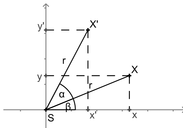
Obrázek 11: Otočení \mathcal{R}([0, 0], \alpha)
