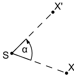
Obrázek 10: Otočení \mathcal{R}(S, \alpha)
