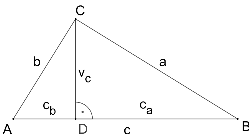
Obrázek 8: Eukleidovy Základy, Kniha VI., Tvrzení VIII.
