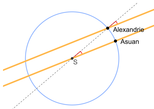
Obrázek 11: Eratosthenovo měření obvodu Země
