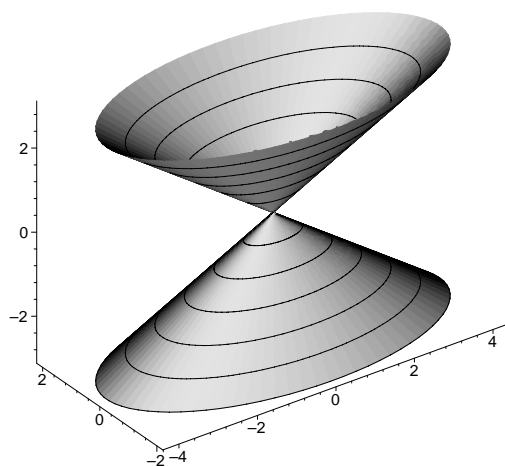
Obrázek 2.36: Kuželová plocha
