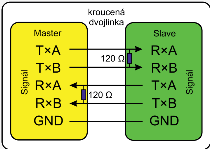
Obrázek: Blokové schéma RS422 - signály
